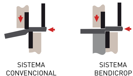
3 Sistema antitorsión para corte de llantas sin deformación.
